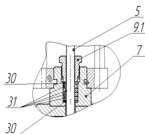
Рисунок 4. Сальниковый узел.
