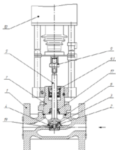
Рисунок 2. Незагруженный по давлению клапан DN 15 – 40. Исполнение А.
