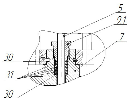
Рисунок 4. Сальниковый узел.
