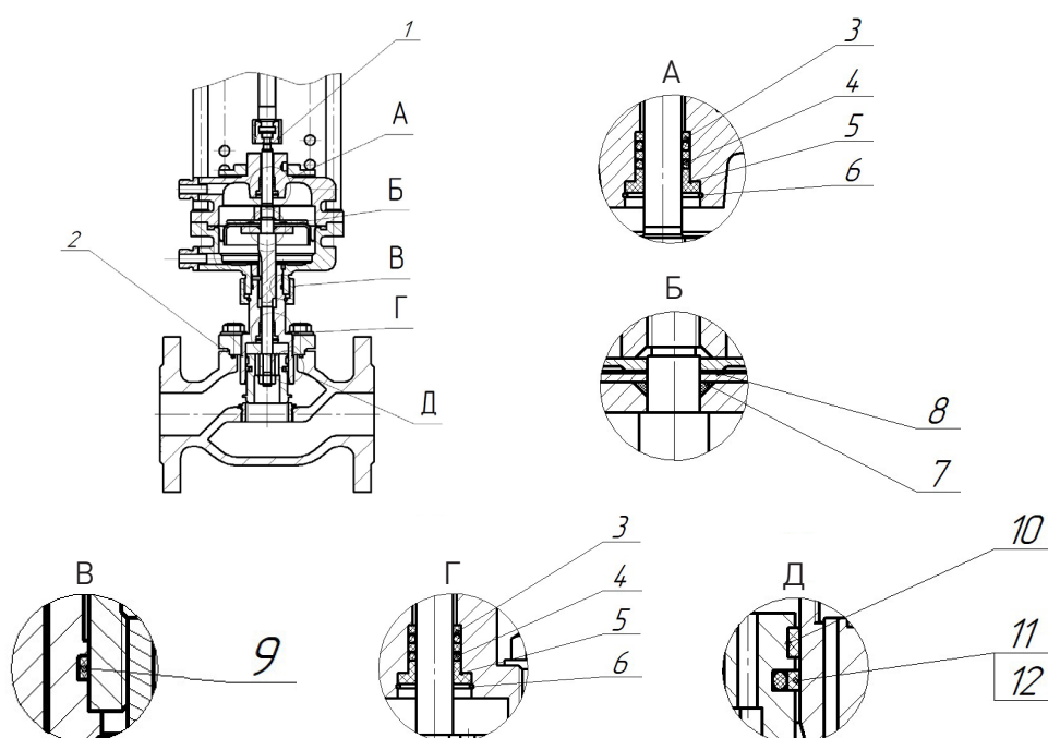
Рисунок 5. Ремкомплекты.
