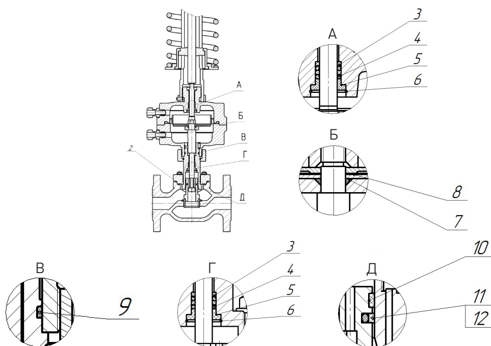
Рисунок 5. Ремкомплекты.
