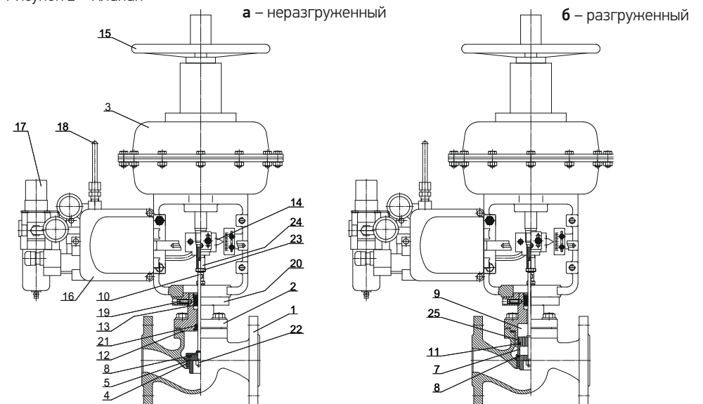
Рисунок 2 – Клапан
